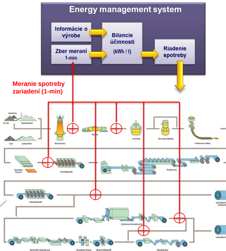
Schéma výrobného procesu
